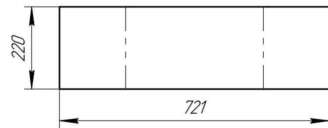
Дет. поз. 2 (1:2,5)
