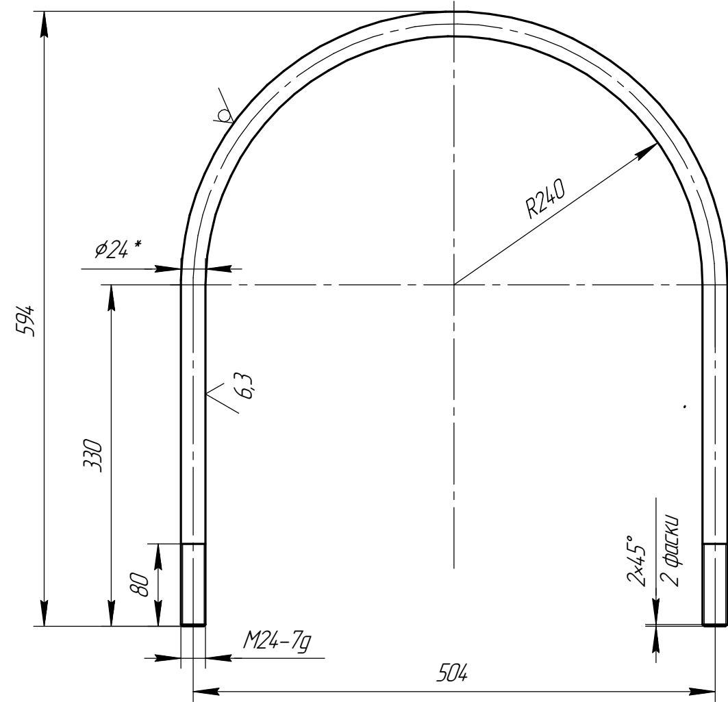
Дет. поз. 5 (1:5)
