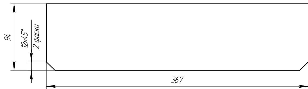
Дет. поз. 2 (1:2,5)
